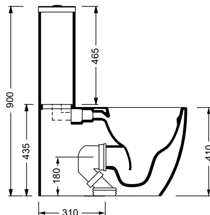
Con connessione traslata per scarico a suolo. ACS 102 With outlying drainage connector for floor trap. ACS 102
