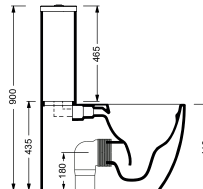
Con connessione per scarico a suolo regolabile. ACS 103 With adjustable drainage connector for floor trap. ACS 103
