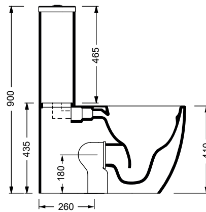
Con connessione per scarico a suolo. ACS 100 With drainage connector for floor trap. ACS 100
